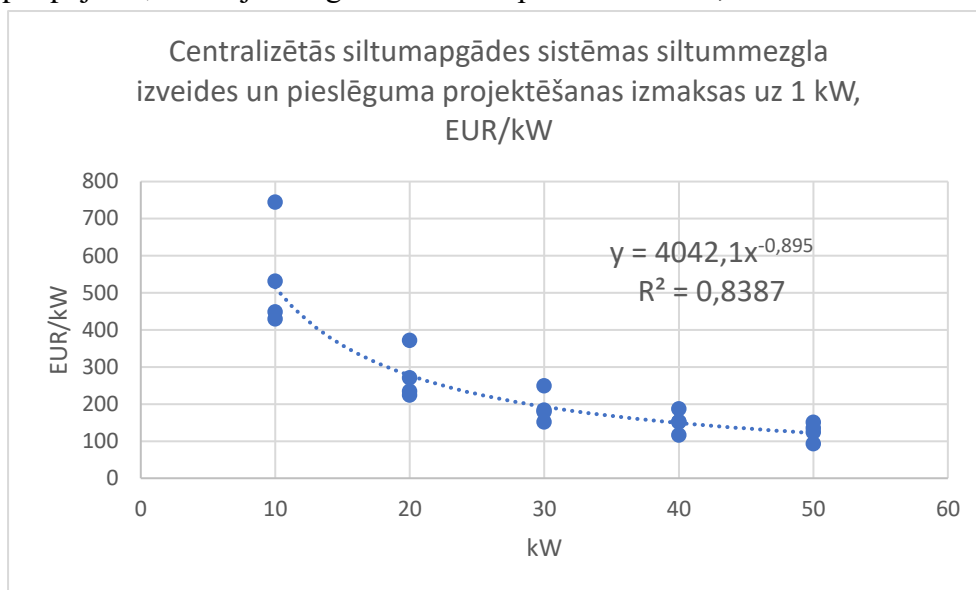
5.attēls. Centralizētas siltumapgādes sistēmas siltummezgla izveides un pieslēguma projektēšanas izmaksu apkopojums, funkcijas un grafiskais attēls 78 .
