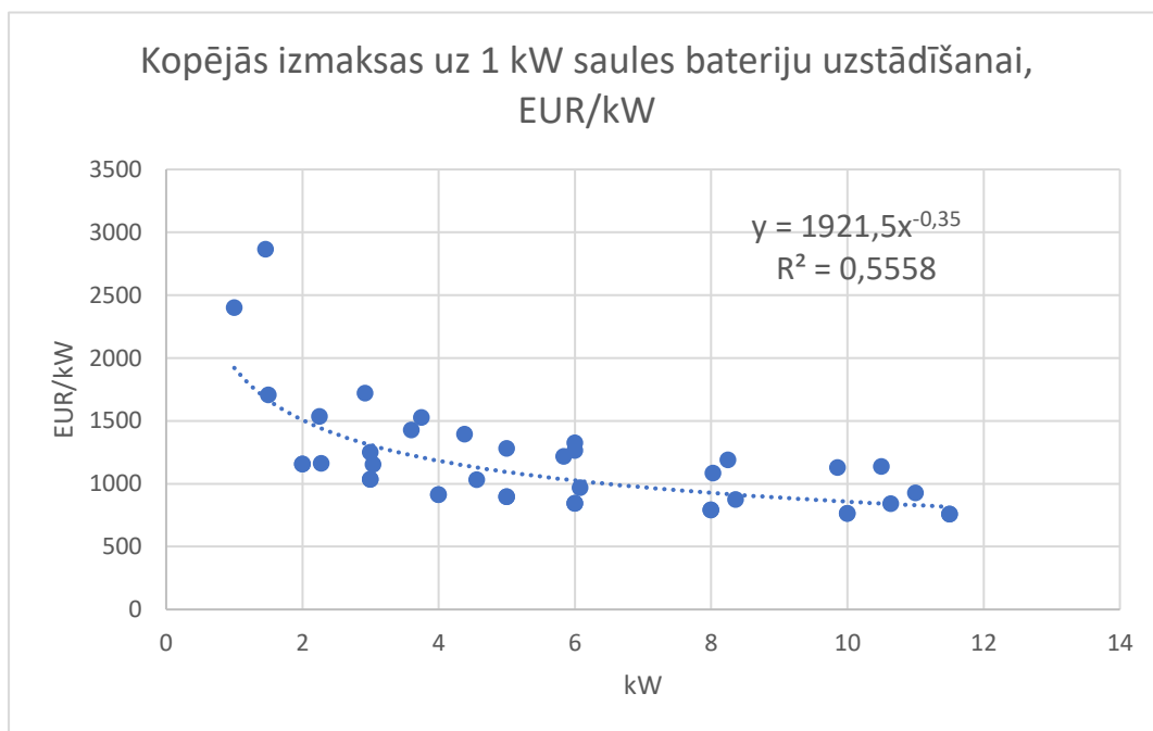
9.attēls Saules paneļu sistēmas ar pieslēgumu elektrotīklam iegādes, uzstādīšanas un ierīkošanas izmaksu apkopojums, funkcijas un grafiskais attēls 88 .
