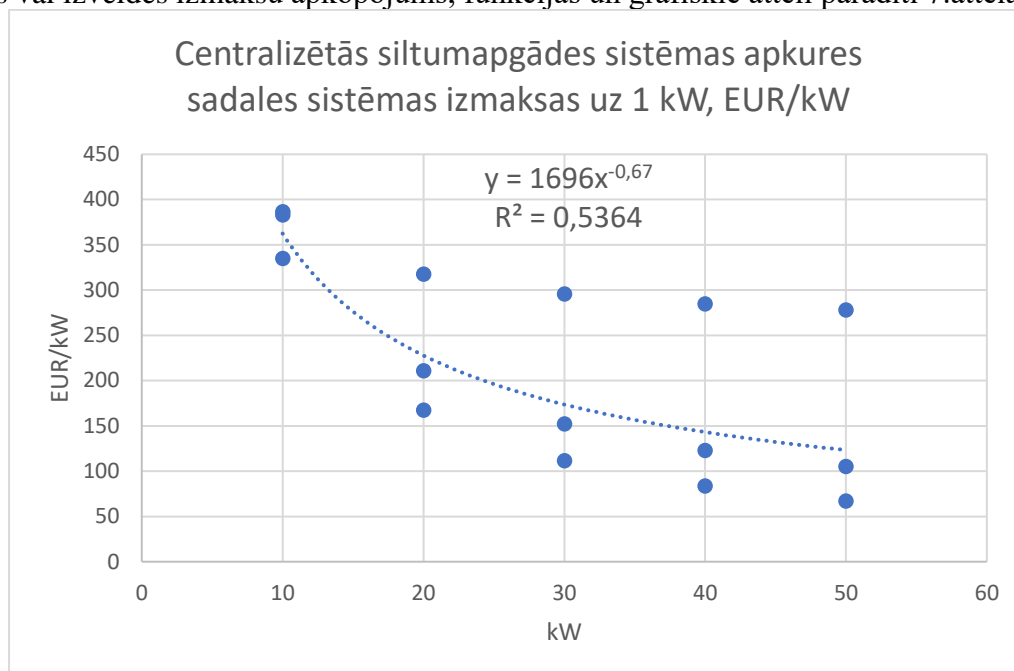
7.attēls. Centralizētas siltumapgādes sistēmas apkures sadales sistēmas pilnīgas atjaunošanas, pārbūves vai izveides izmaksu apkopojums, funkcijas un grafiskais attēls 80 .
