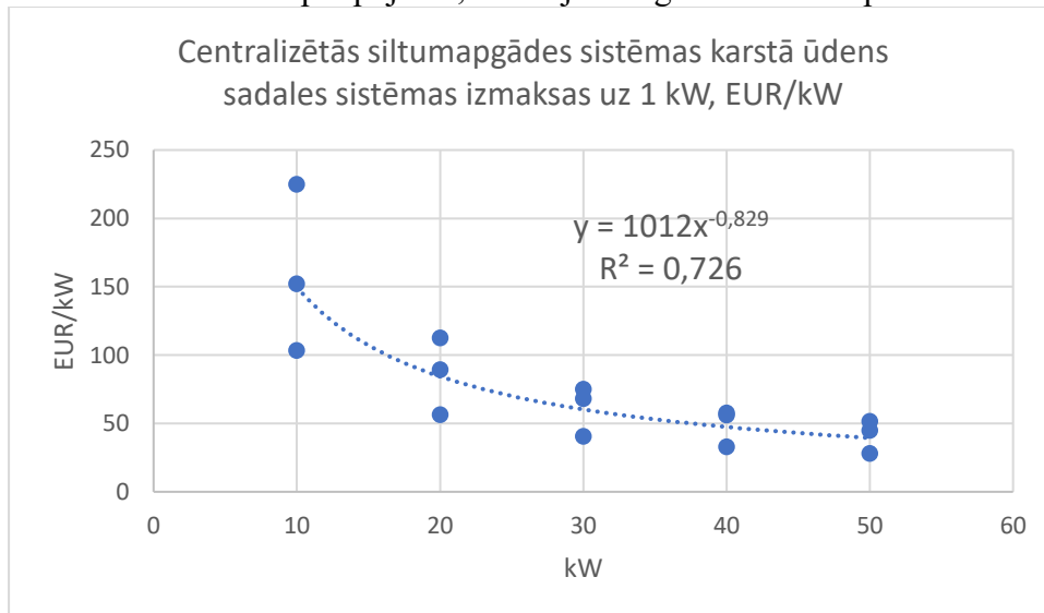
6.attēls. Centralizētas siltumapgādes sistēmas karstā ūdens sadales sistēmas pilnīgas atjaunošanas, pārbūves vai izveides izmaksu apkopojums, funkcijas un grafiskais attēls 79 .
