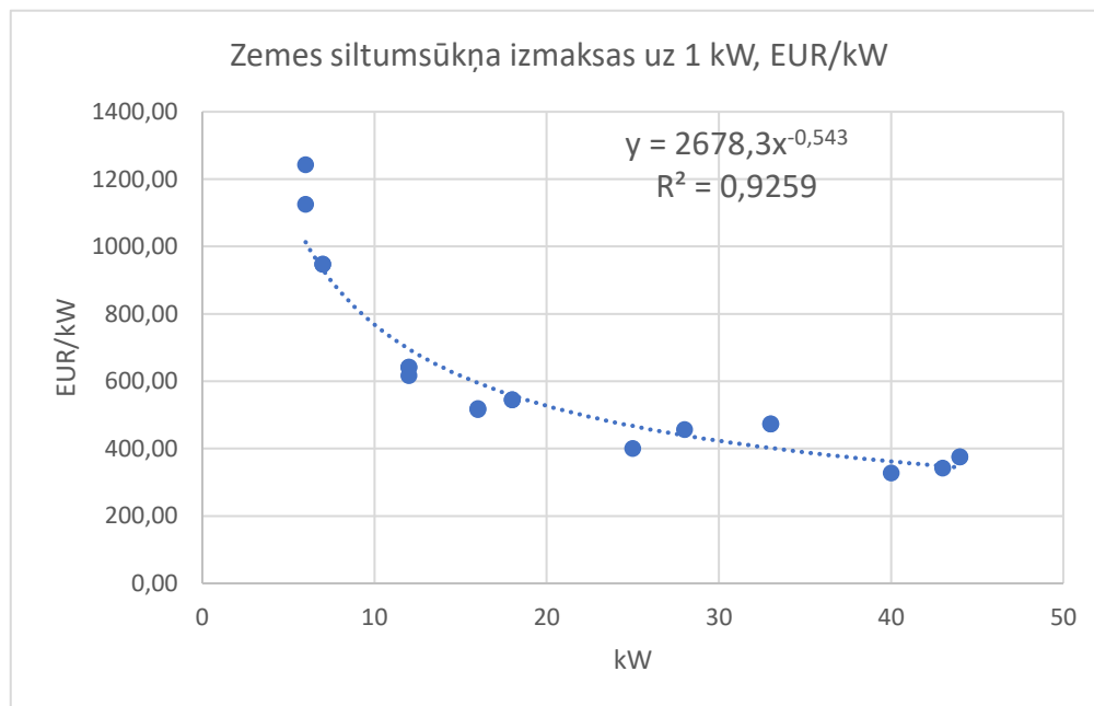
2.attēls. Zeme-ūdens tipa siltumsūkņu izmaksu apkopojums, funkcijas un grafiskais attēls 73 .
