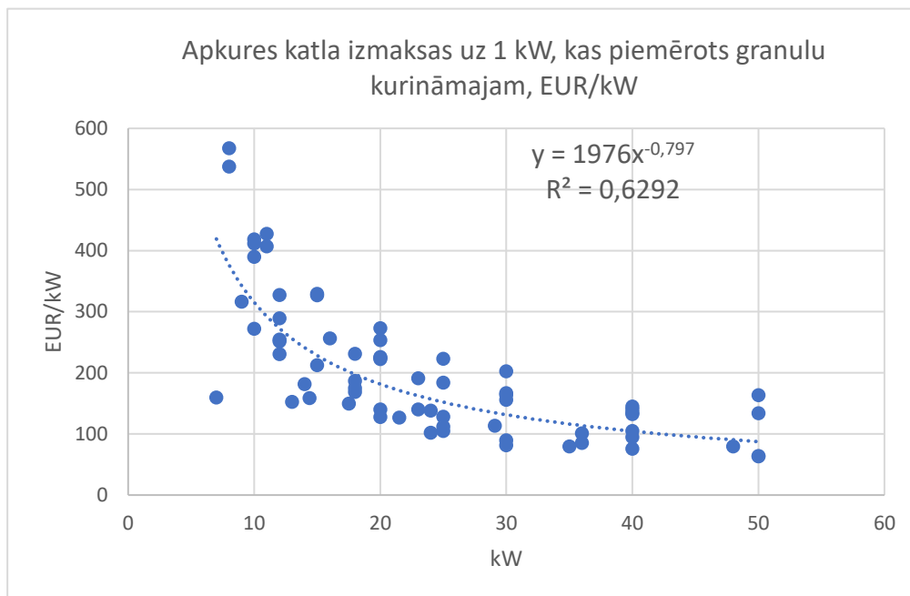
1.attēls. Koksnes biomasas apkures katlu, kas piemēroti granulu kurināmajam, izmaksu apkopojums, funkcijas un grafiskais attēls 72 .
