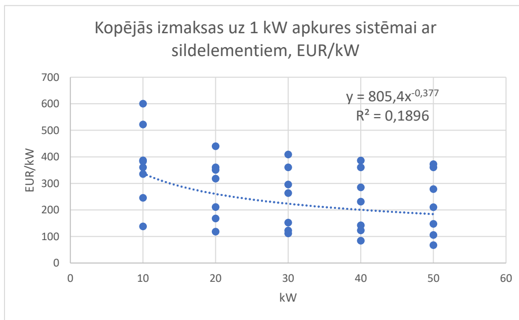
8.attēls. apkures sistēmas ar sildelementiem pilnīgas atjaunošanas, pārbūves vai izveides sistēmu izmaksu apkopojums, funkcijas un grafiskais attēls 82 .
